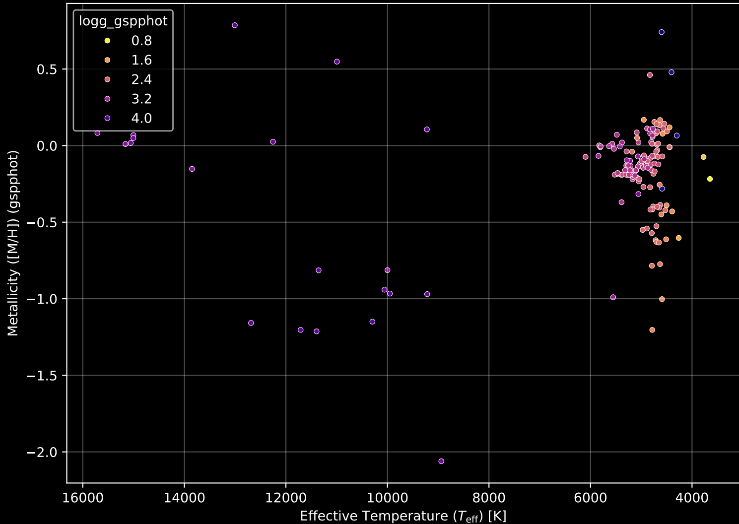
APOGEE DR17 Field: [229+04] Stellar Population Parameters (n= 160)
